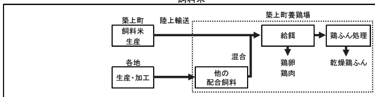
第1図 トウモロコシ飼料および飼料米のシステム境界の設定
